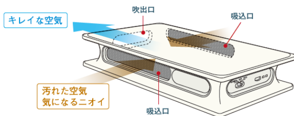
図2：「全周風道設計」による空気の流れ
