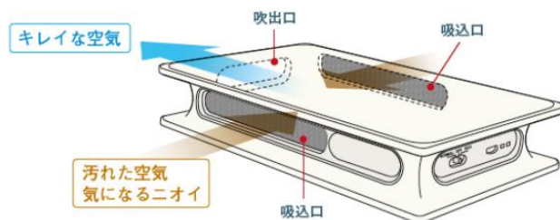
図2：「全周風道設計」による空気の流れ
